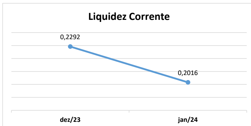
Gráfico 2: Liquidez Corrente
